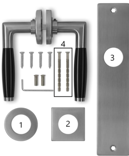
Afb.1 Onderdelen
