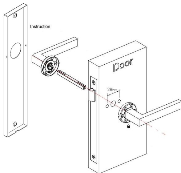
Afb.2 Montagevolgorde
