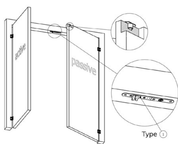
Deze naar binnendraaiende passieve deur is DIN rechts
