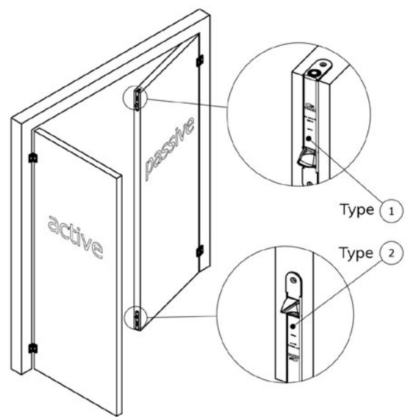
Deze naar binnendraaiende passieve deur is DIN rechts
