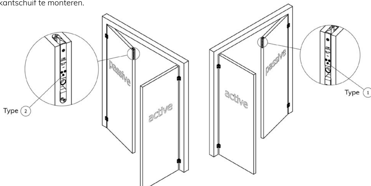
Deze naar binnendraaiende passieve deur is DIN links
