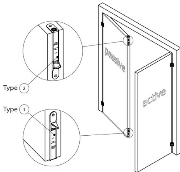
Deze naar binnendraaiende passieve deur is DIN Links
