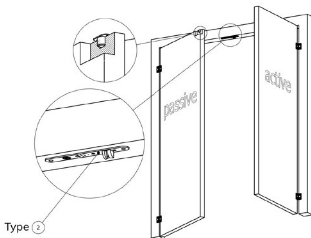
Deze naar binnendraaiende passieve deur is DIN links
